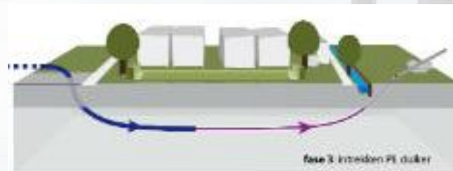
Fase 3: buis erin trekken
